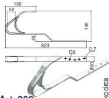
Art. 399 Gancio sottotegola Under roof tile hook
